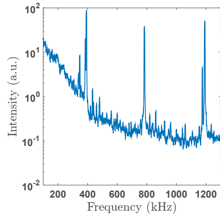
(d) Cathode power spectrum. B = 1.5 B^*
